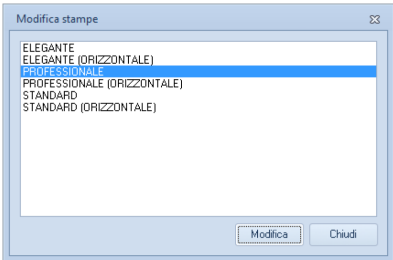
Modifica stampe
