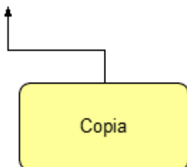
Copia
