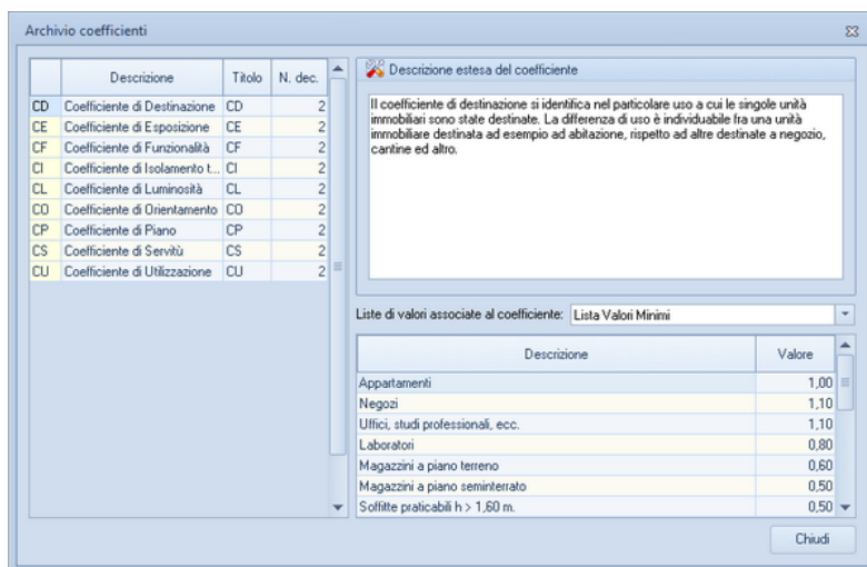
Archivio coefficienti
