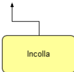
Incolla
