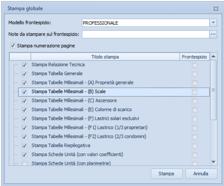
Stampa Globale
