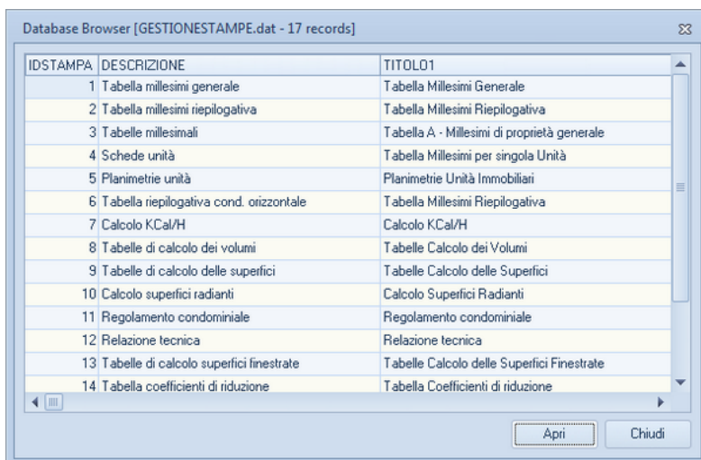
Database browser
