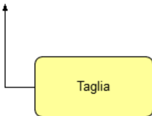
Taglia
